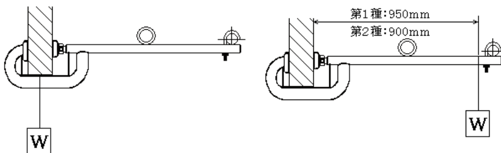
取り付け部の滑り ( 締め付けトルク 530kg/cm )
