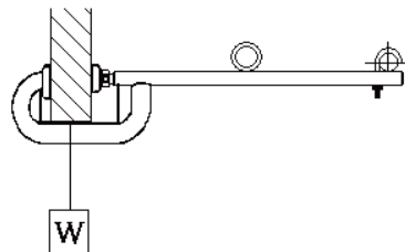
取り付け部の滑り（締め付けトルク 530kg/cm）
