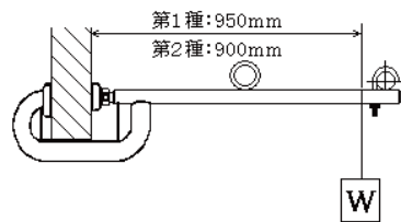
ポストのたわみと強度
