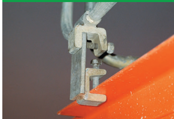
C型鋼用取付金具
