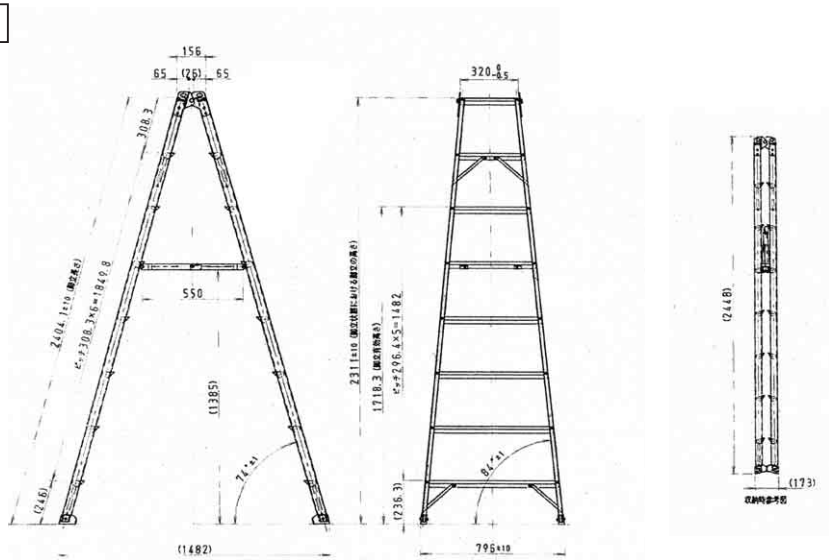
8尺
