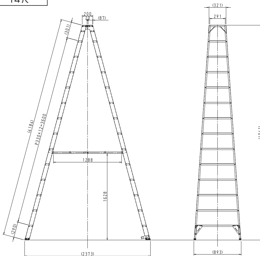
14尺
