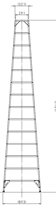
折畳参考図
